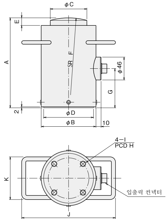
CLP-1~5MNB
